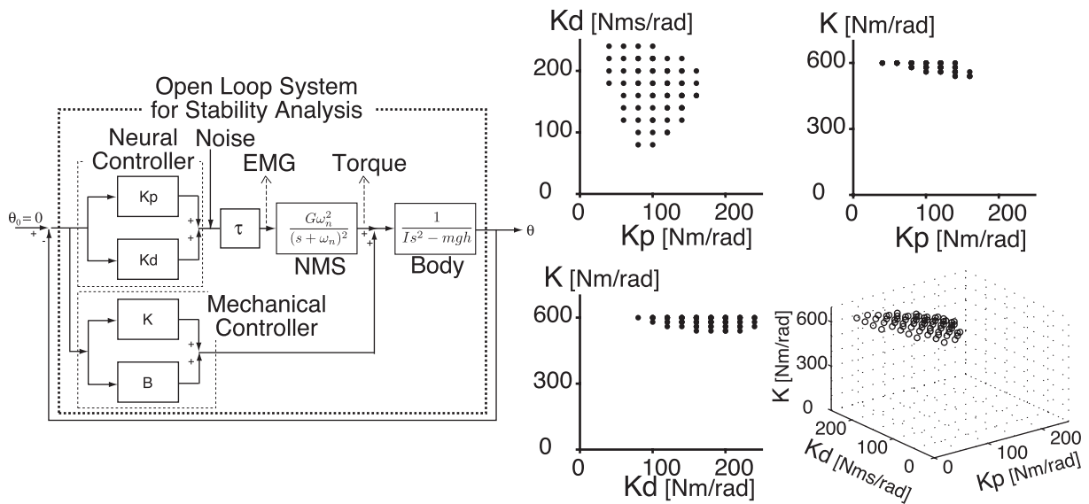
図3 立位制御系のモデル (左) とシミュレーションに用いたゲインセット (右)。左: 立位制御系モデルは, 神経系制御器 (Neural Controller), 粘弾性 (Mechanical Controller), 神経-筋系 (NMS), 身体に相当する倒立振子 (Body), 伝達時間遅れ ( \tau ) から成る。太点線で囲まれた領域を安定性解析に用いた。右: 各ゲインは, 神経系比例ゲイン ( K_p ), 神経系微分ゲイン ( K_d ), 弾性 ( K ), 粘性 ( B = 5 \text{ Nms/rad} ) を表す。安定性解析で安定と判定されたゲインセットを3次元プロットした (右下)。この3次元プロットを K_p - K_d 面 (左上), K_p - K 面 (右上), K_d - K 面 (左下) に投射した図も付した。
