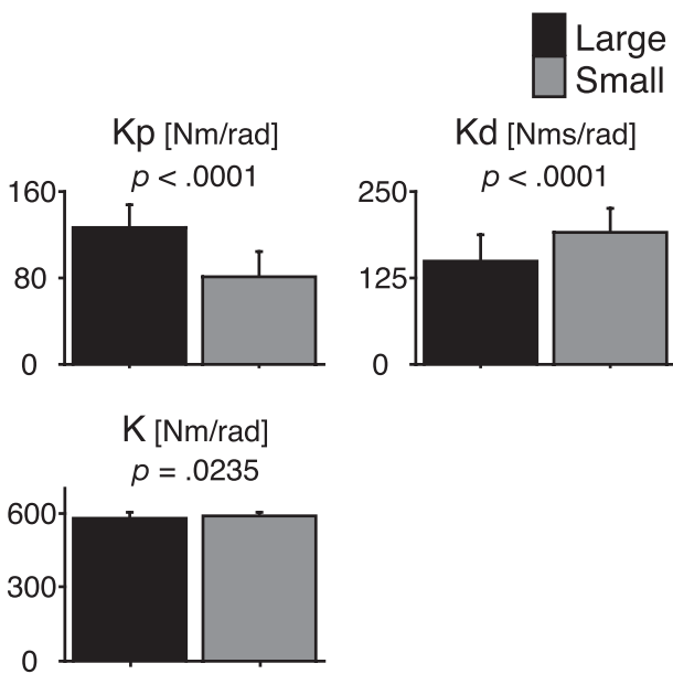
図6 シミュレーションで得られた Large 群 (高齢者相当) と Small 群 (若齢者相当) のゲインセットの比較. 左上: 神経系比例ゲイン (Kp), 右上: 神経系微分ゲイン (Kd), 左下: 弾性 (K) のそれぞれを Large 群と Small 群について示した. p 値は両群平均値の差についての t 検定結果を表す.
