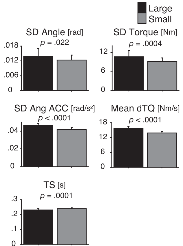
図5 シミュレーションで得られた Large 群（高齢者相当）と Small 群（若齢者相当）の身体動揺各評価変数の比較。各略字はそれぞれ身体重心角変位の標準偏差（SD Angle）、足関節トルク変動の標準偏差（SD Torque）、身体重心角加速度の標準偏差（SD Ang ACC）、足関節トルクの一階微分系列平均振幅（Mean dTQ）、運動指令の身体重心変位に対する先行時間（TS）を表す。p 値は両群平均値の差についての t 検定結果を表す。
