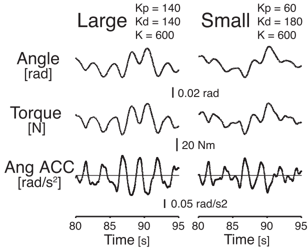
図4 シミュレーションで得られた Large 群（高齢者相当）と Small 群（若齢者相当）の身体動揺。上から、身体重心角変位、足関節トルク変動、身体重心角加速度 (Ang ACC) を表す。
